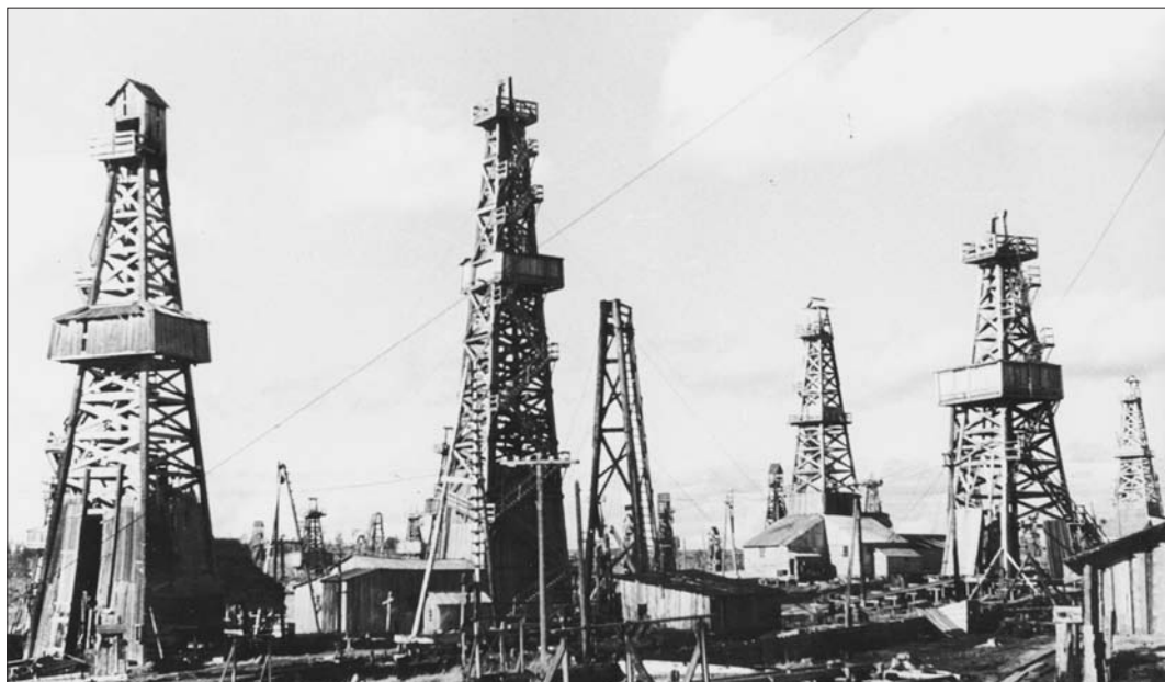
Ил. 5. Общий вид Охинского нефтепромысла. 1937 г. Фотограф Прехнер. ГИАСО. Фотофонд. Оп. 1. Ед. хр. 4909
