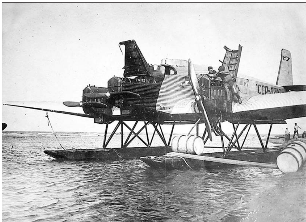
Ил. 9. Гидросамолет «Юнкерс», использовавшийся для связи Северного Сахалина с материком
